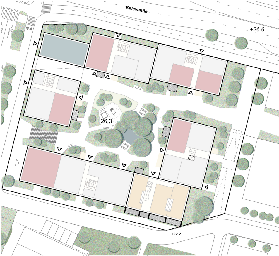
Kansi- / Kalevantien taso n. +26,3 1:800
