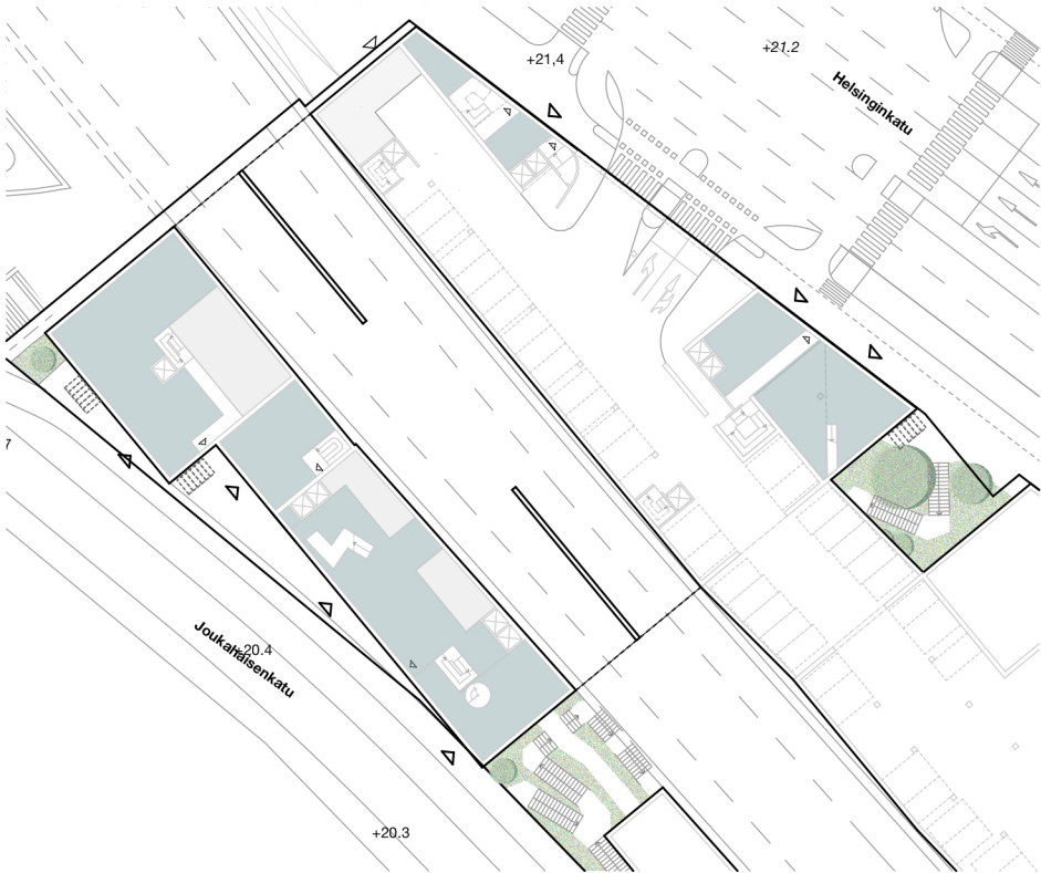
Katutaso n. +21,4 1:900
