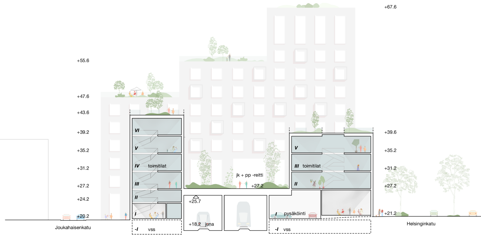
Leikkaus aa 1:500
