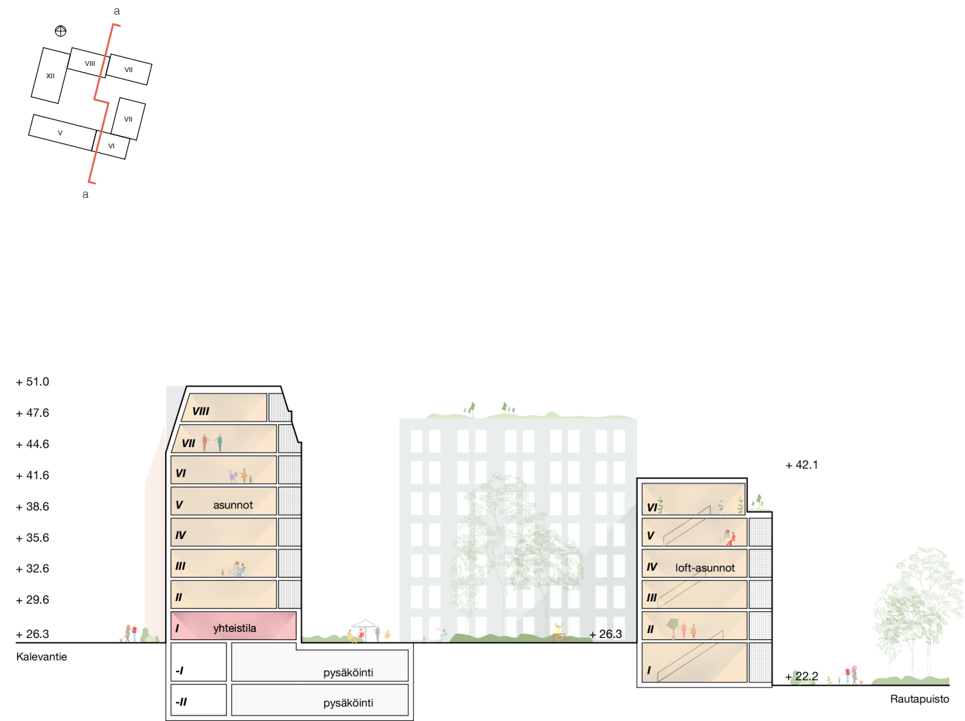
Leikkaus aa 1:500
