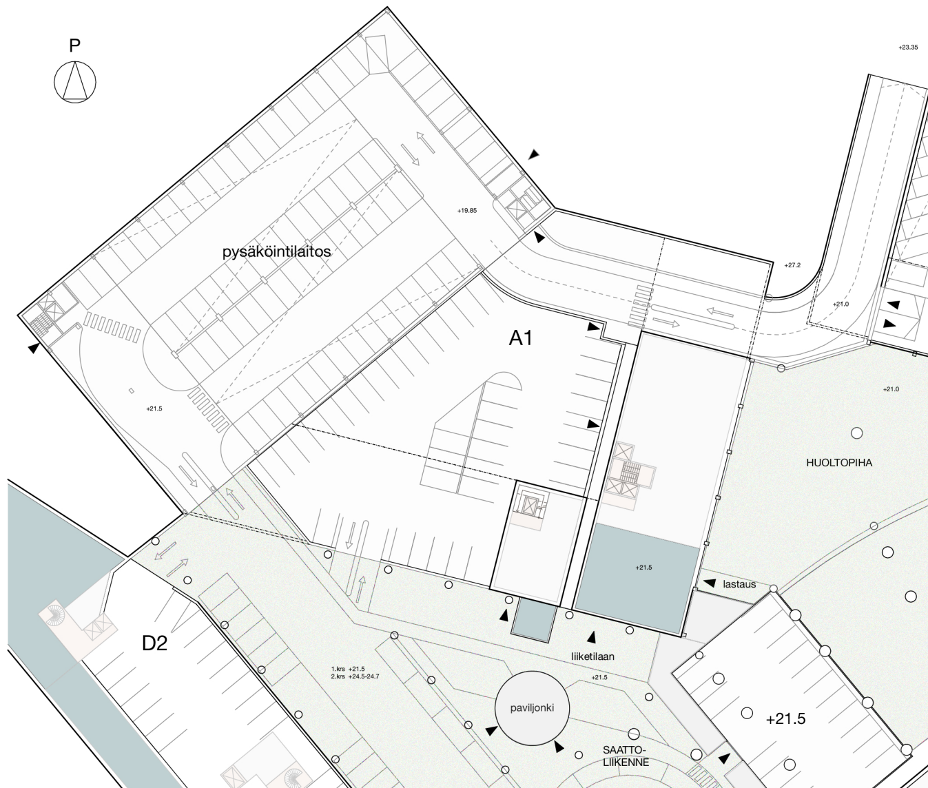
Katutaso n. +21,5 1:700
