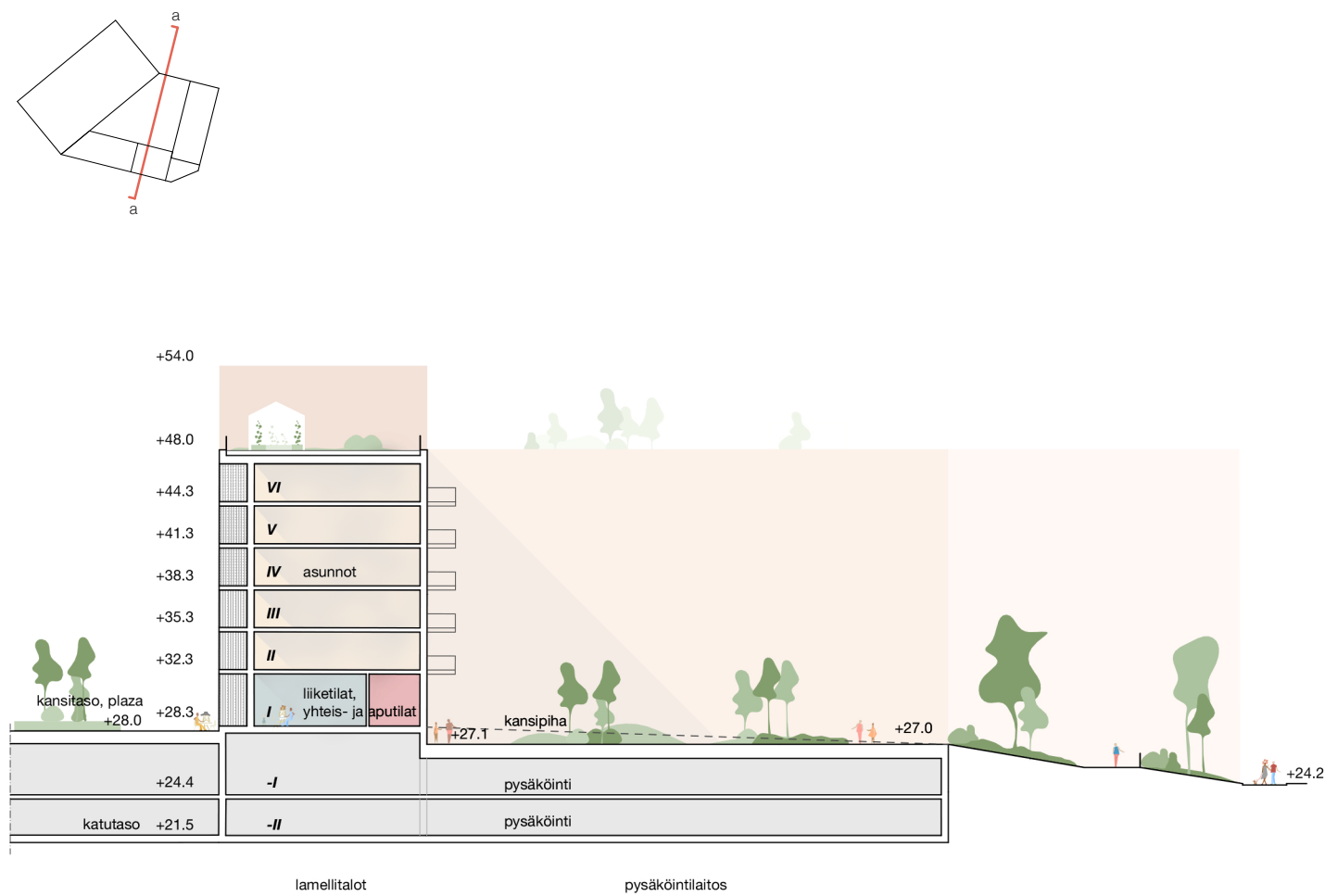
Leikkaus aa 1:500
