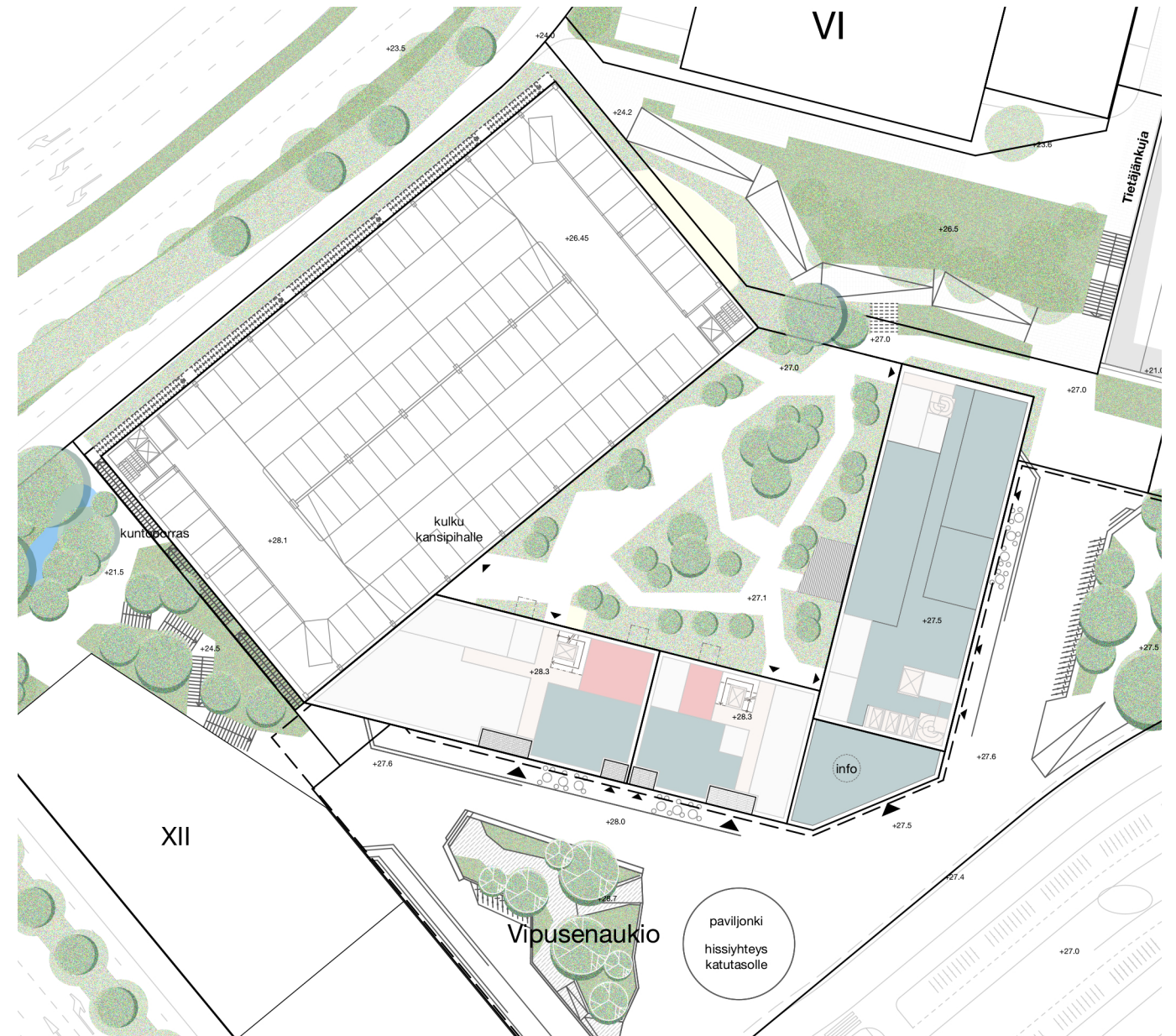
Kansitaso n. +27,5...+28,0 1:700
