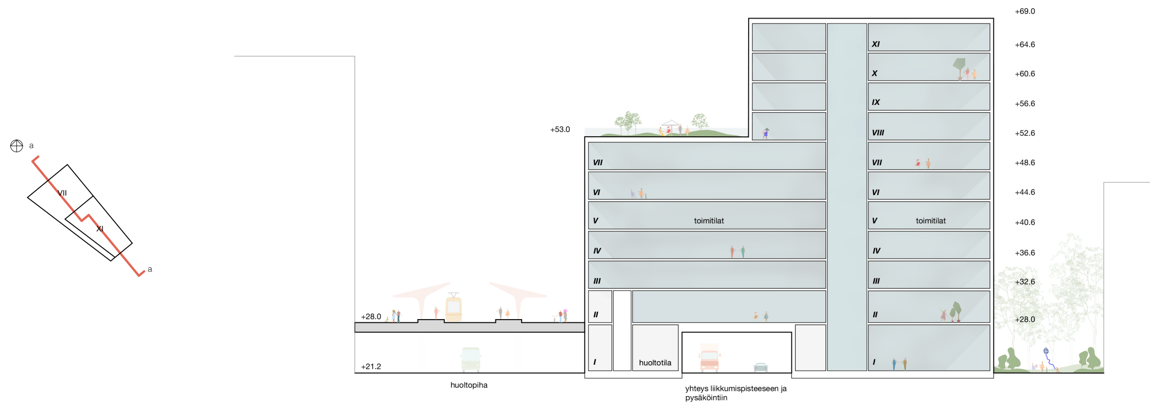
Pitkittäisleikkaus 1:500
