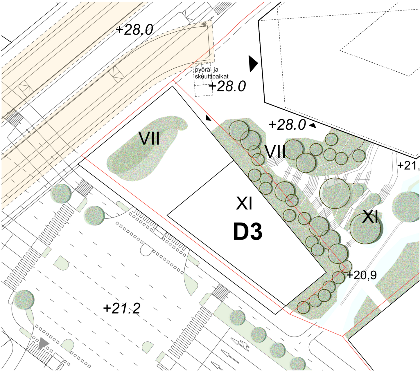
Pihapiirustus 1:500
