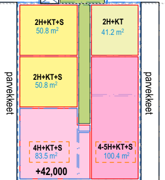
7.kerros
