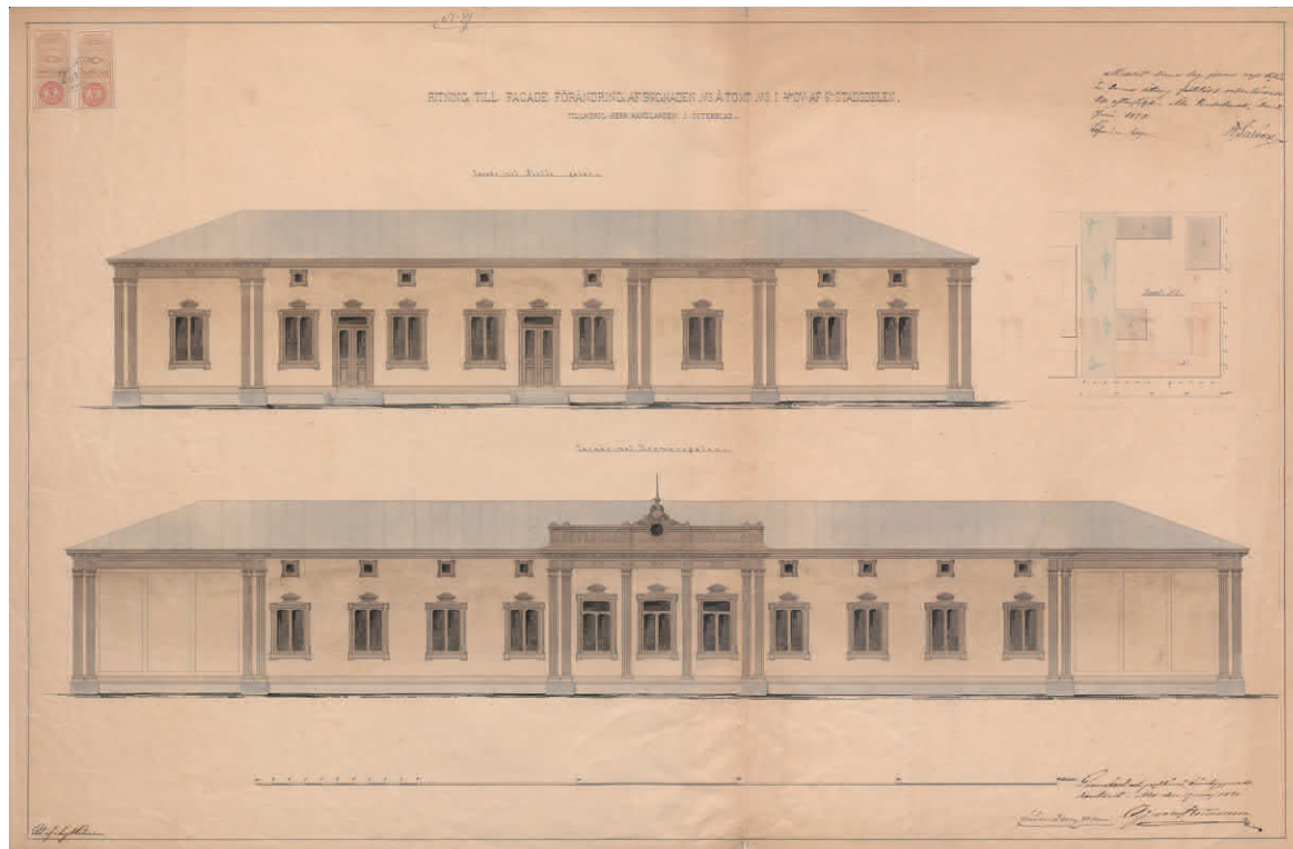
Linnan- ja Kauppiaskatujen kulmauksen rakennuksen julkisivut uudistettiin uusrenessanssityyliseksi vuonna 1880. KA Turku, TMPP.
