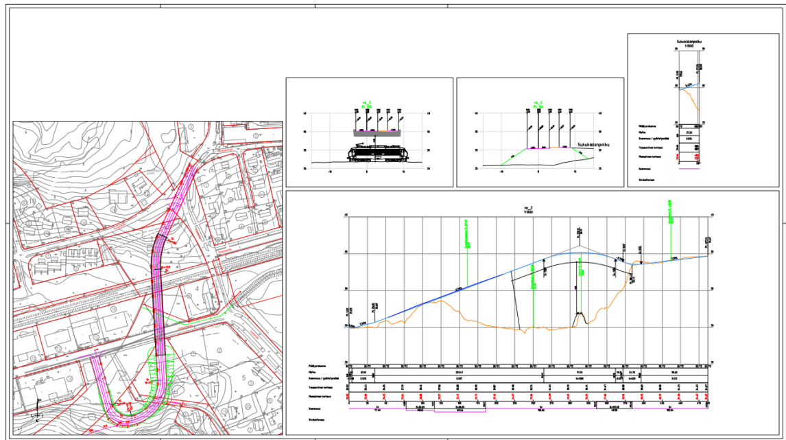
Kuva 16. Esiselvitysvaiheen suunnitelma ylittävstä vaihtoehdosta 15.5.2020.
