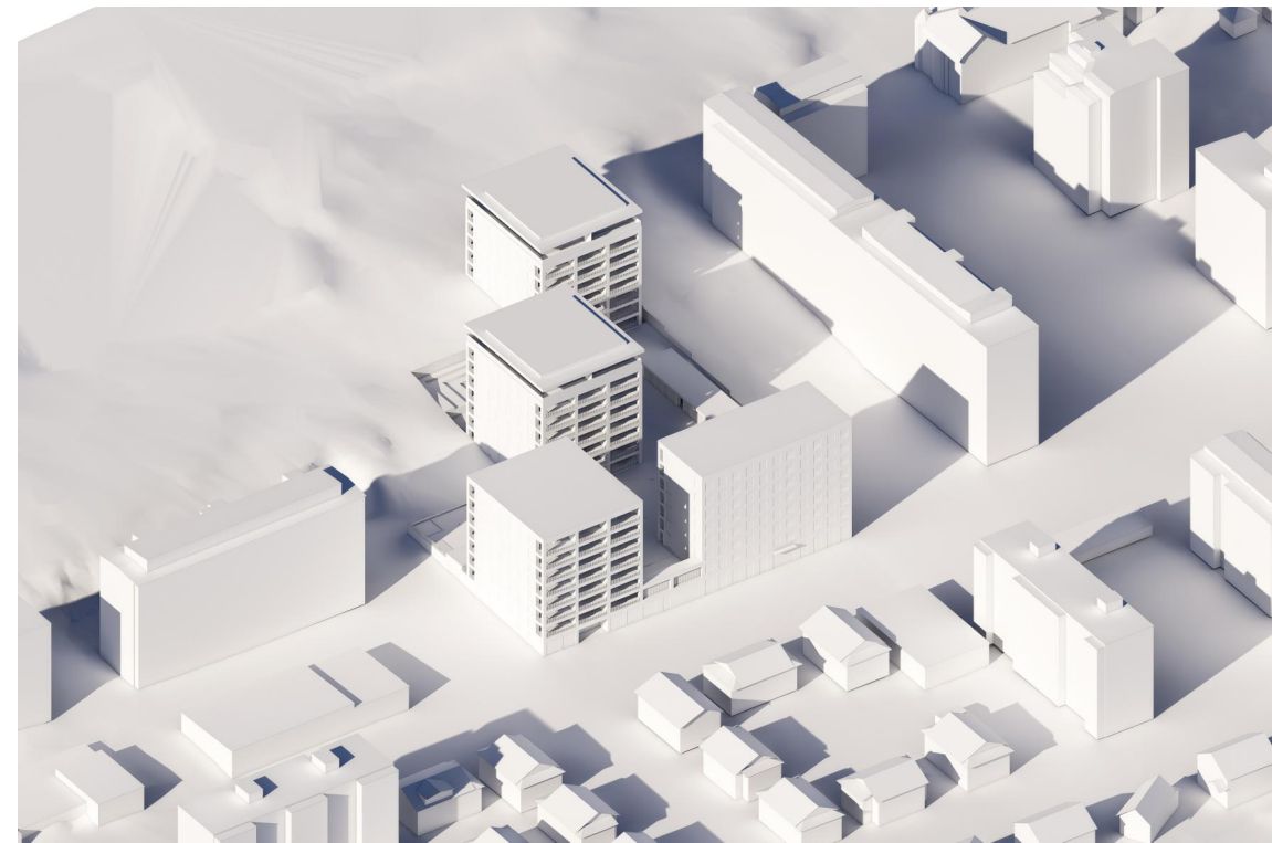
Kevätpäiväntasaus klo 14
