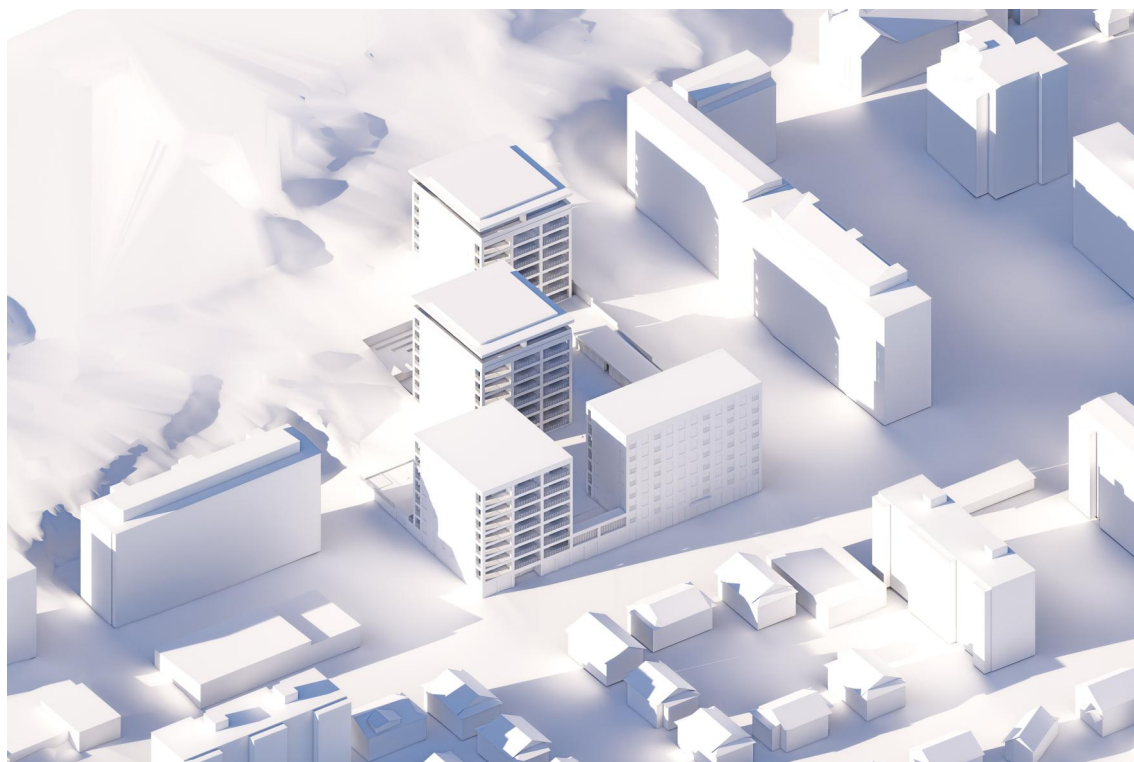
Kevätpäiväntasaus klo 16
