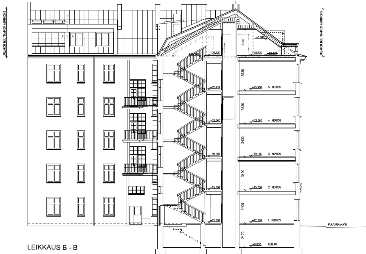
Kuva 2. Alustava suunnitelma ullakkorakentamisesta osoitteessa Puutarhakatku 16. Leikkauspiirustus ei mittakaavassa. (20.1.2023, Haroma & Partners Arkkitehtitoimisto).
