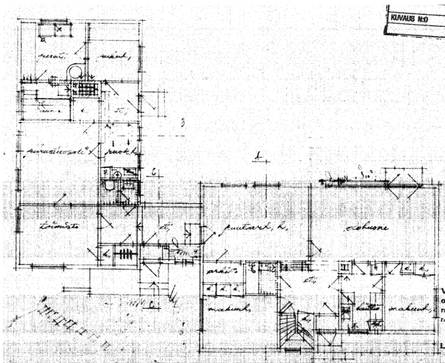
Asunnon ja toimiston pohjakuva, rakennuslupakuva 1952 (TKA). Keskellä olevasta nivelosasta on käynti sekä siiven toimistotiloihin että asuinrakennuksen kulkussa olevaan puutarhurin työhuoneeseen.
