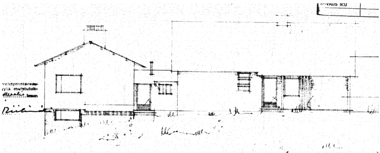
Päärakennuksen julkisivut Uudenmaantien suuntaan, rakennuslupakuva 1952 (TKA). Asunto oikealla ja toimistorakennuksen pääty vasemmalla.
