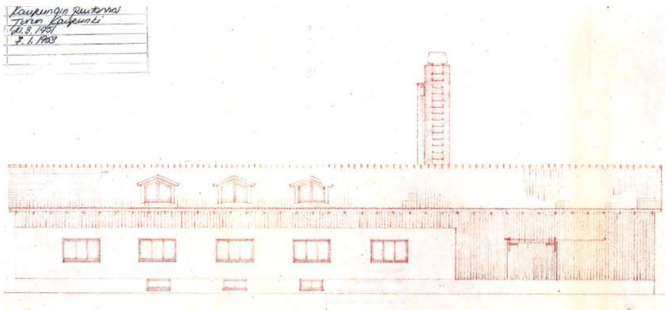
Kasvihuoneiden yhdysrakennuksen julkisivu Uudenmaantielle, lupakuva 1951 (RakVa).
