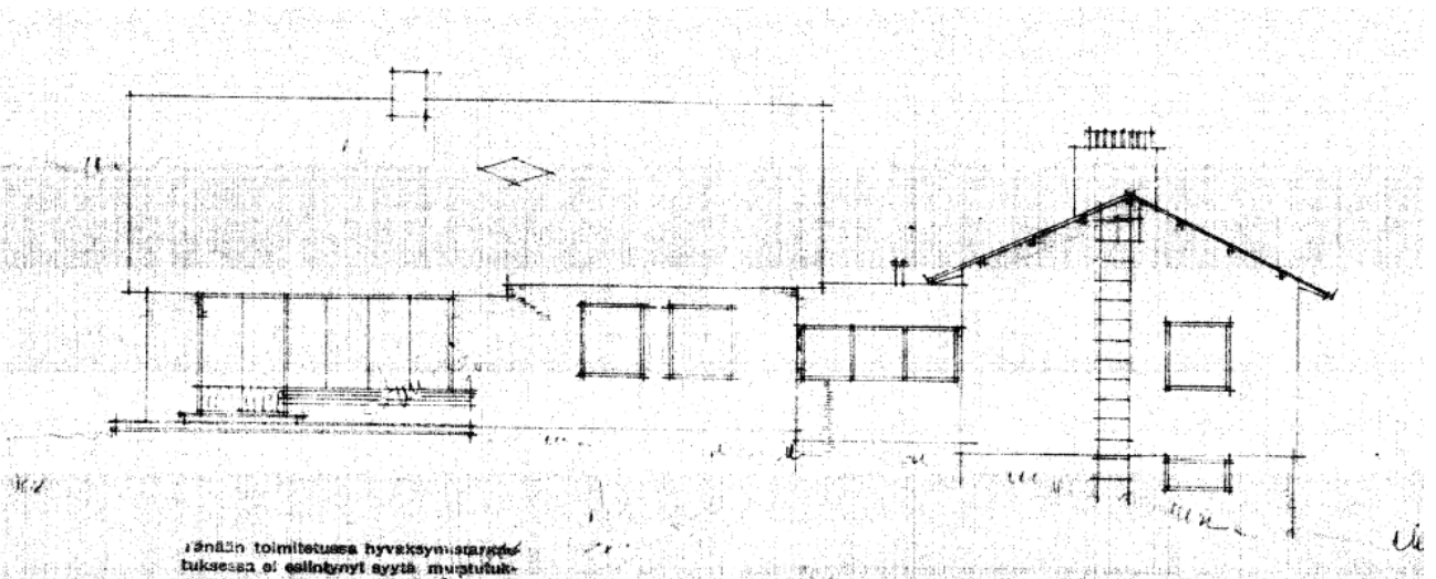
Julkisivut Ruiskadun suuntaan, rakennuslupakuva 1952 (TKA). Asunto vasemmalla ja toimistorakennuksen pääty oikealla.
