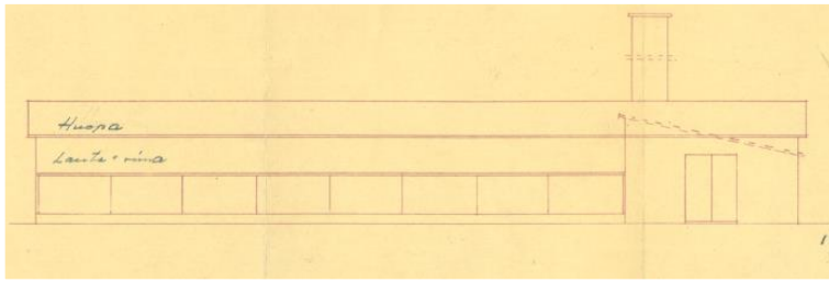
Suunnitelma vanhimpien kasvihuoneiden lämpökeskuksen muutoksesta 1950 (SRK). Vanha huoltorakennus oli jätetty pystyyn kattilahuoneen ja sen yläpuolisen työhuoneen osalta. Rakennus oli aiemmin ollut Ilpoistentien suuntainen, nyt se muutettiin Uudenmaantien suuntaiseksi.
