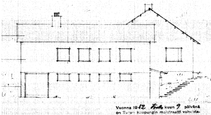
Toimistorakennuksen sivu Ilpoistentien suuntaan, taustalla asuinrakennuksen pääty. Rakennuslupakuva 1952 (TKA).
