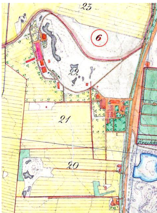
Tiluslohkot 20–23 vuoden 1930 mittauskartalla (KYTO, paikkatieto ja kaupunkimittaus). Kartalla näkyy seurakuntien puutarhan uudisrakennukset sekä palstan laajeneminen lohkojen 20, 21 ja 22 alueille (pohjoisraja merkitsemättä). Kuvan vasemmassa yläkulmassa on Fridhemin kauppapuutarha lohkoilla 21–22. Lohkolla 23 toimi Petreliuksen lastenkoti.
