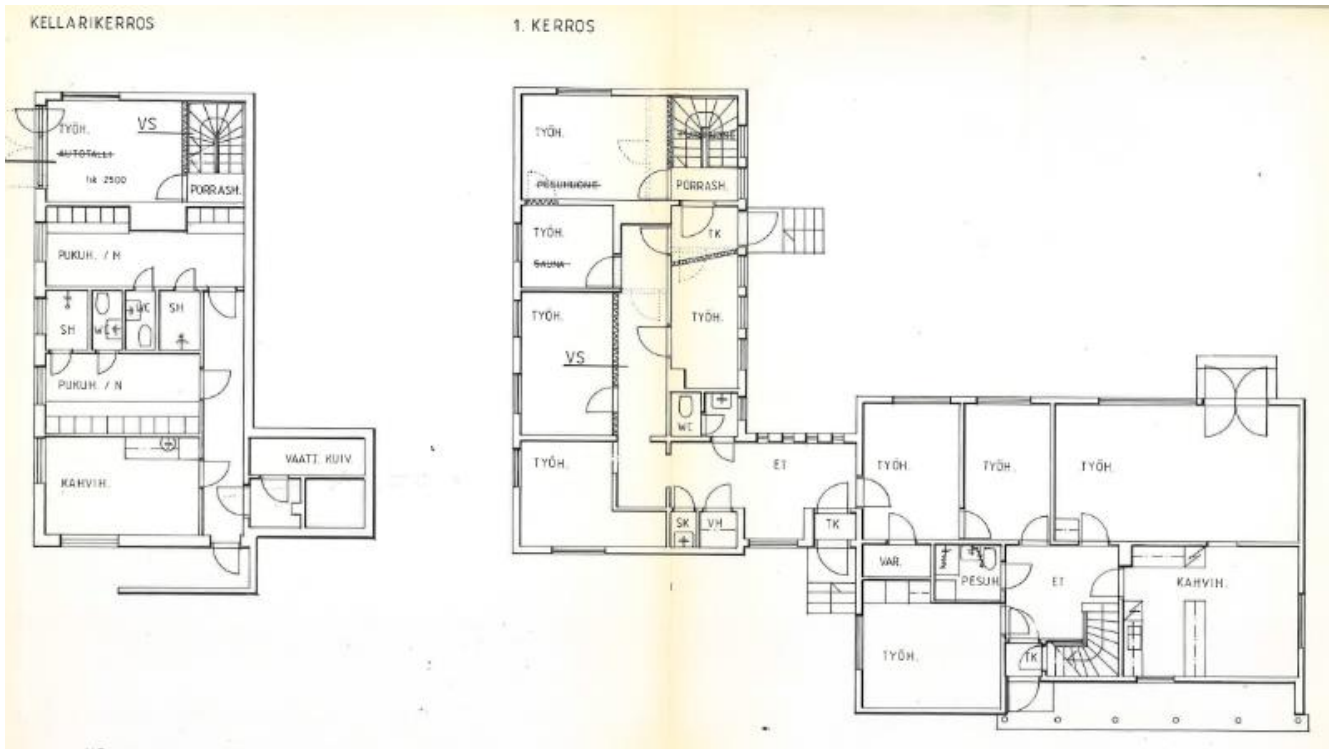
Sisätilojen muutos 1992 (RakVa).
